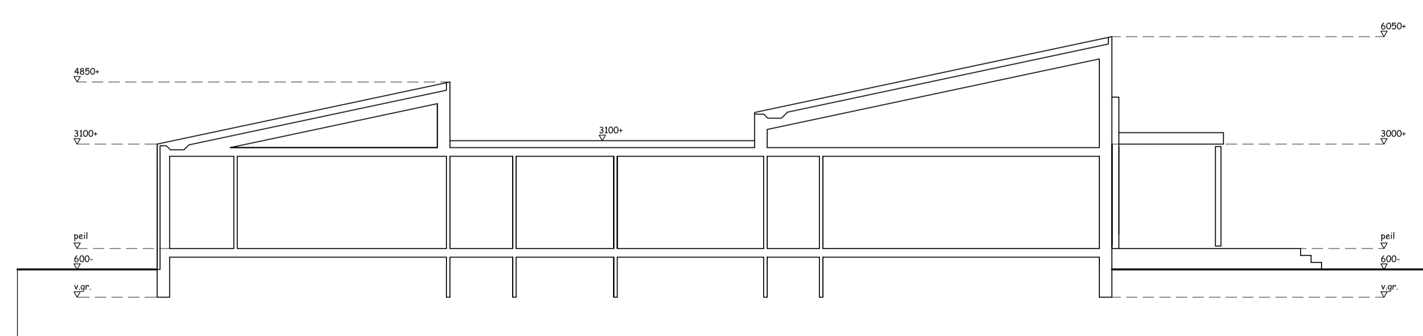
doorsnede a
