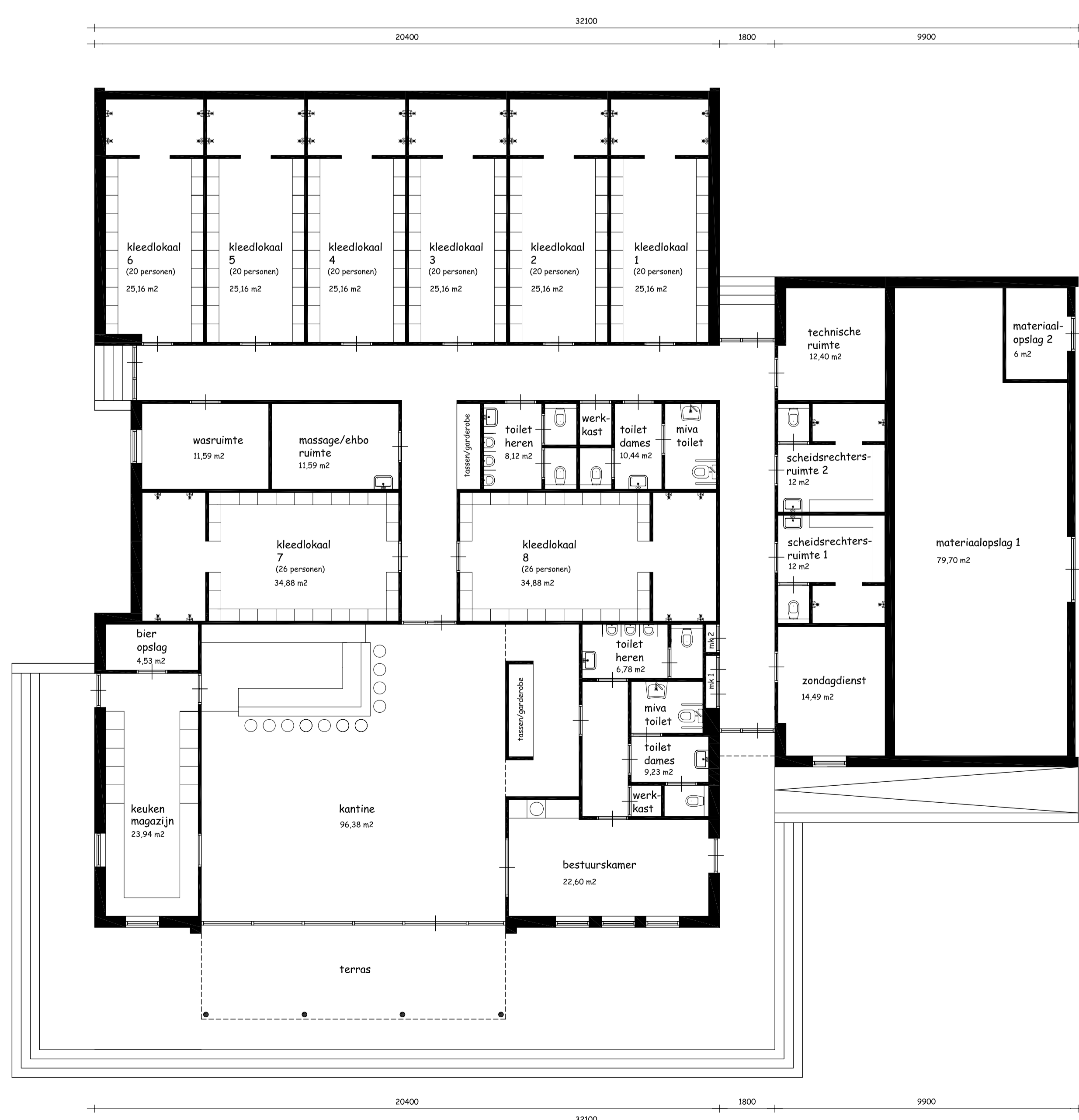
begane grond
